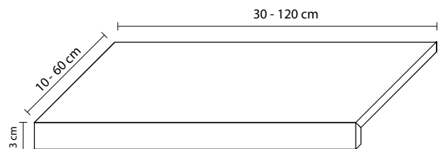
Stufe mit angeklebten Schenkel
