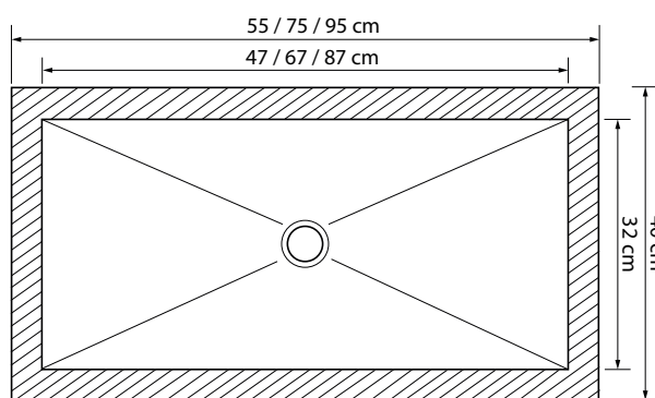
Draufsicht - ohne Abdeckplatte
